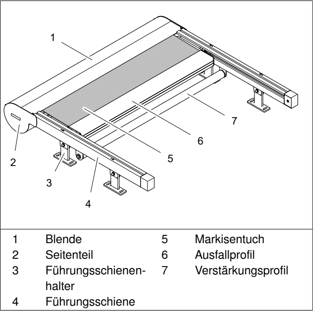
Abb. 1: Teileübersicht Wintergarten-Markise Climara W19
